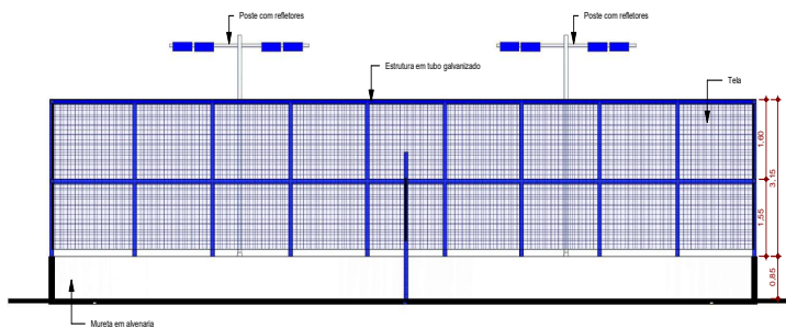
2 CORTE B ESCALA - 1 : 75
