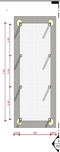
4 PERGOLADO ESCALA - 1 : 75
