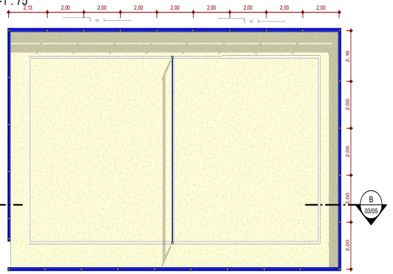
4 PERGOLADO ESCALA - 1 : 75
