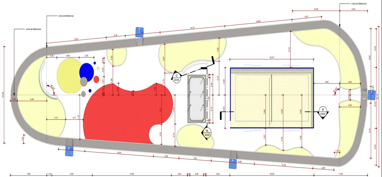
1 PLANTA DE LOCAÇÃO ESCALA -1 : 150
